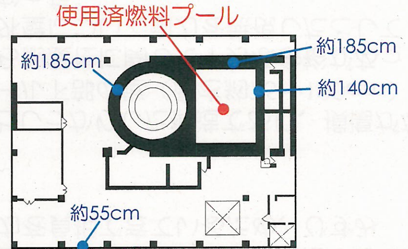
3階 平面図
