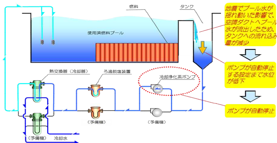
<2-4. 使用済燃料プール冷却浄化系系統図>
