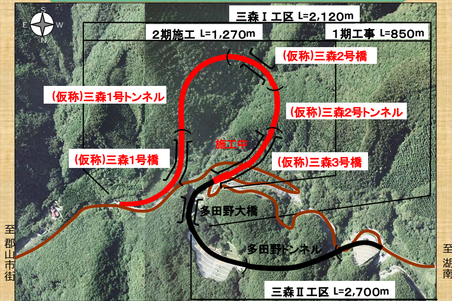
【現場状況 ( (仮称) 三森1号橋) 】 【現場状況 ( (仮称) 三森3号橋) 】
