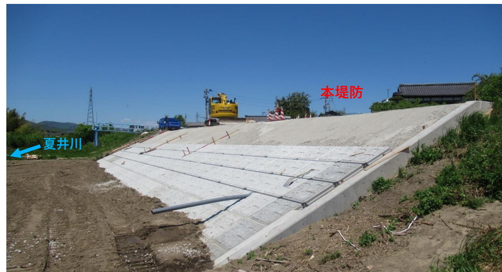
堤防護岸 コンクリート張ブロック施工中 施工状況 (令和2年5月15日)
