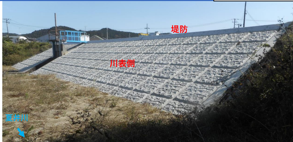
川表側 コンクリート張ブロック完了 (5月末)
