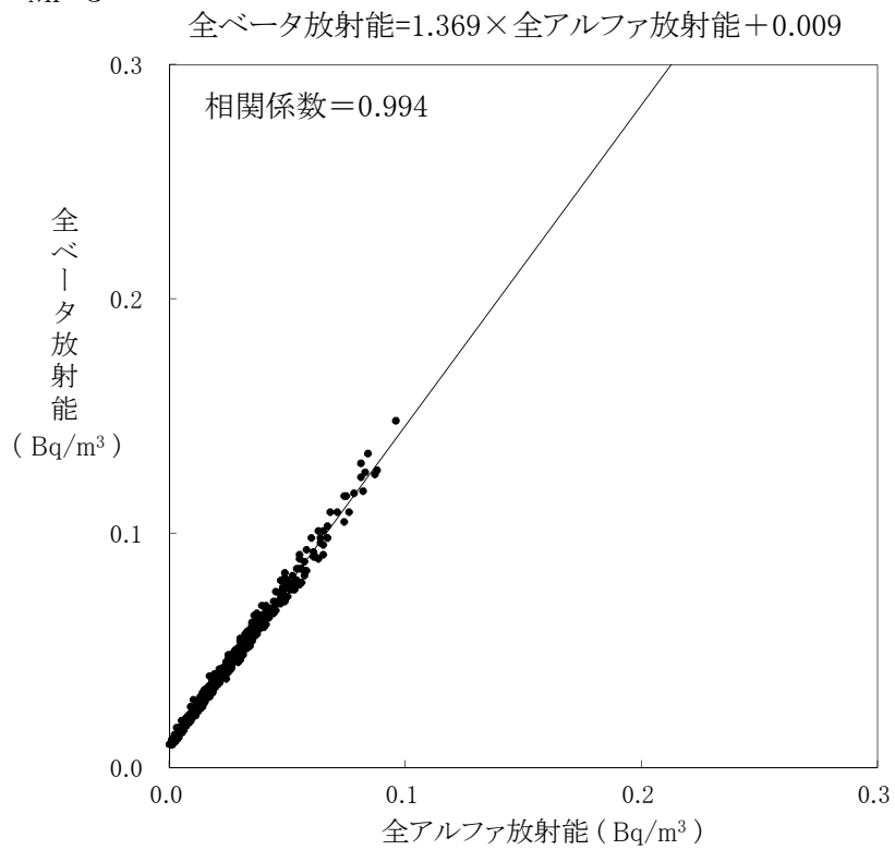
図4.6 全アルファ放射能と全ベータ放射能の相関
