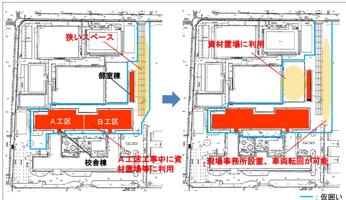
仮設計画図
