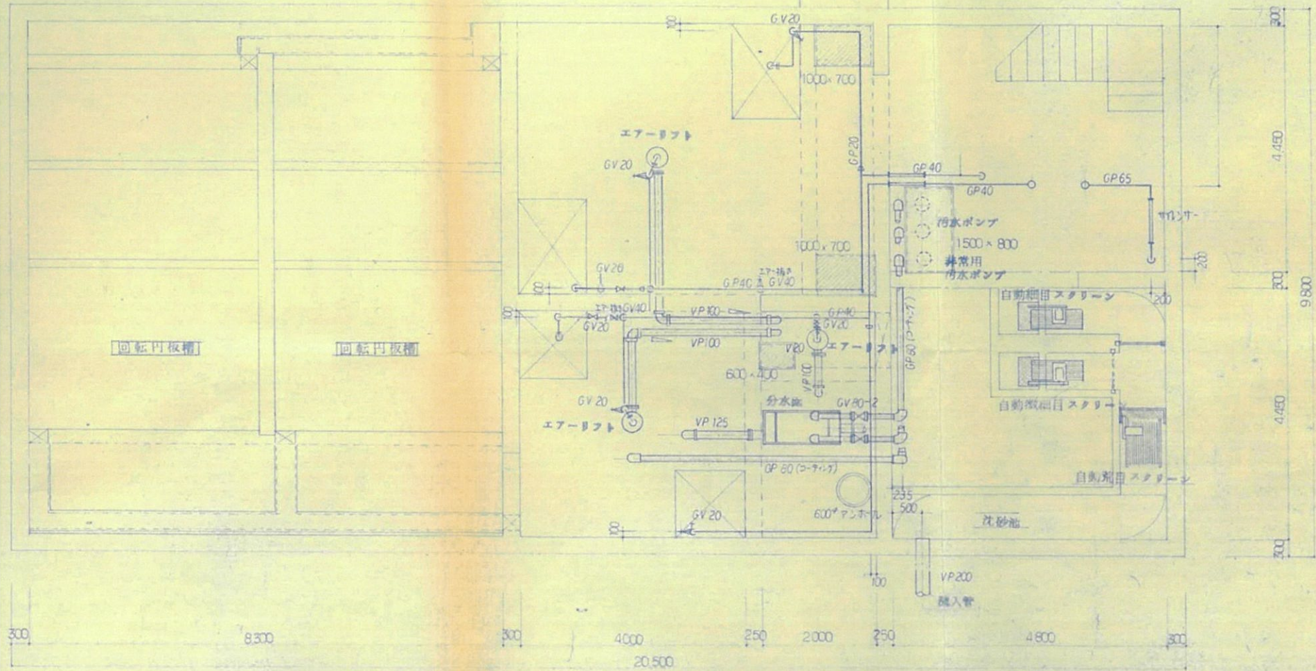
B1 平面図 S=1:60
