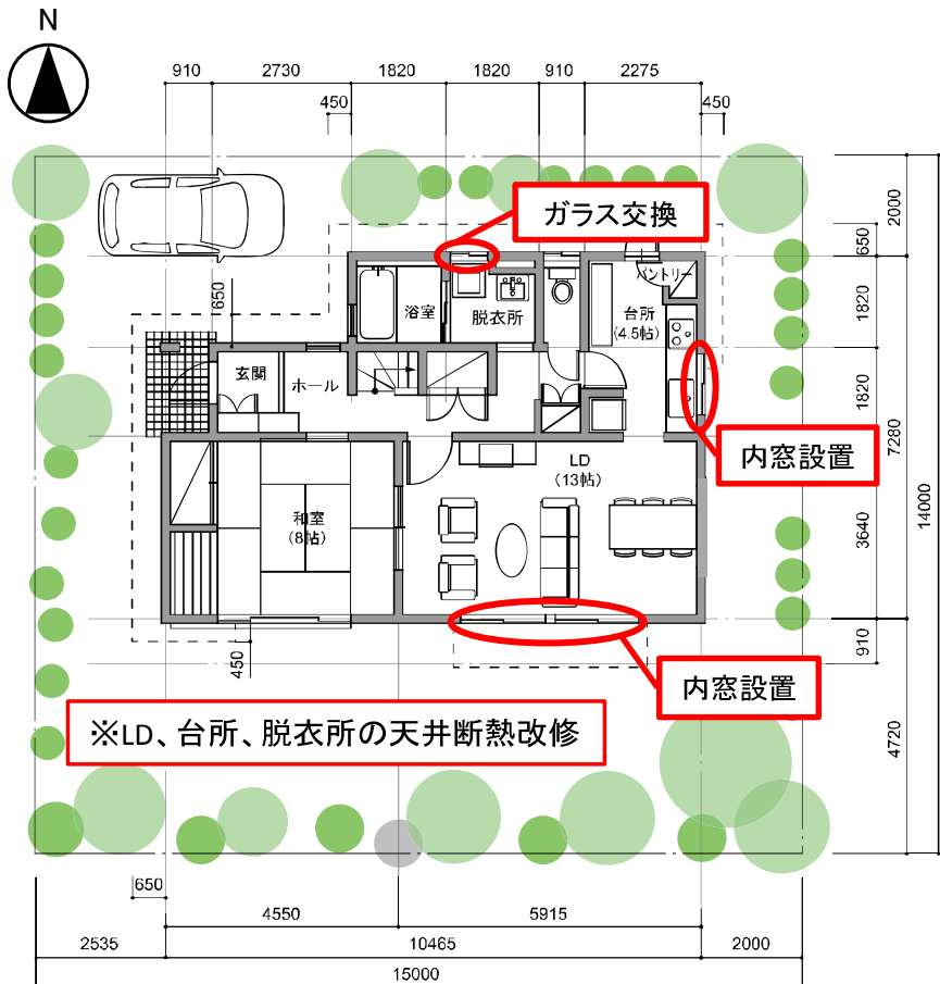
■ 1階平面図
