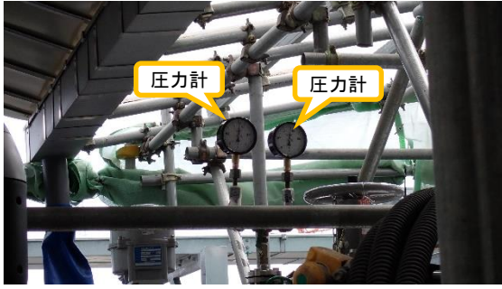
(写真3-1) 圧力の測定状況
