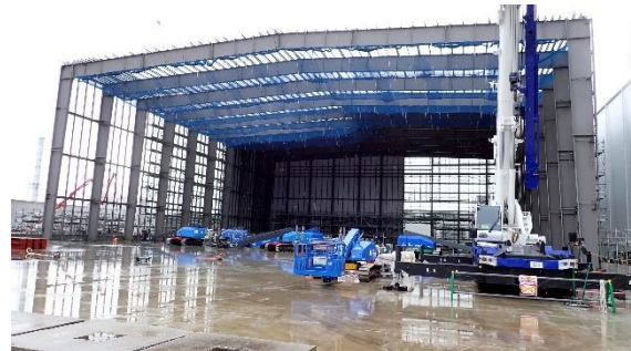
(写真 2 - 2) 固体廃棄物貯蔵庫第 1 0 棟 (B 棟) 建設予定地の状況 (令和 6 年 1 月 2 2 日撮影)
