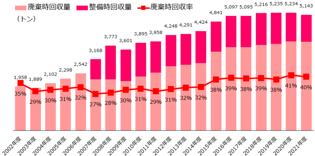
図33 全国の業務用冷凍空調機器からのフロン類回収量等の推移
