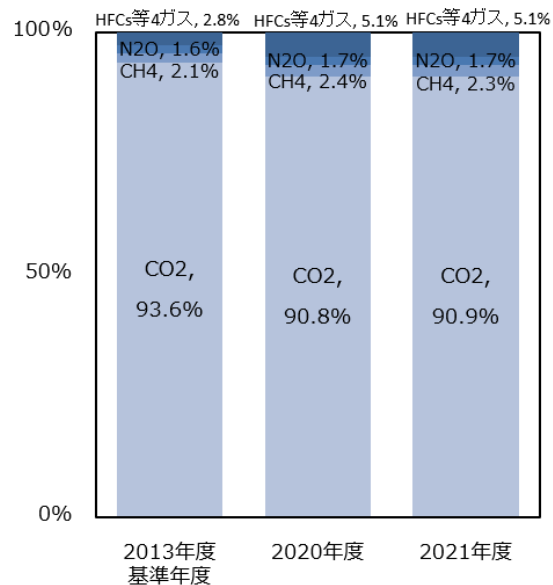
図 7 全国の温室効果ガス排出割合
