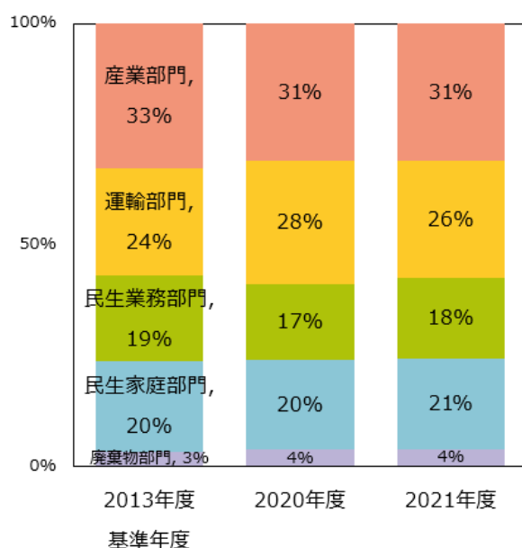
図 9 福島県の部門別二酸化炭素排出割合
