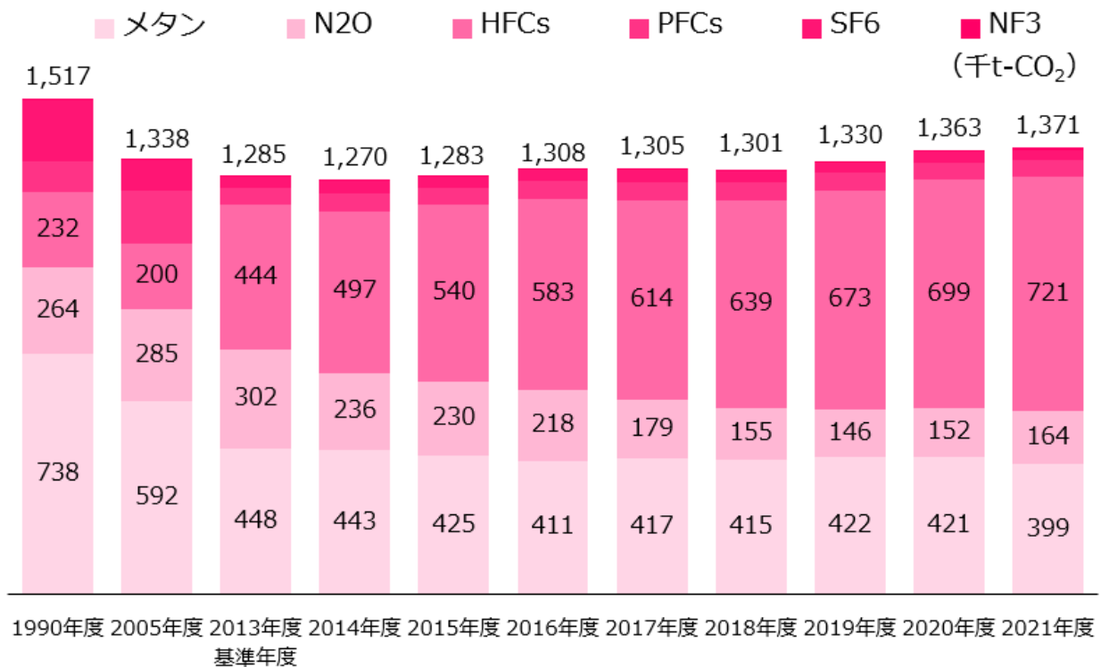
図 29 福島県のその他温室効果ガスの二酸化炭素換算排出量の推移
