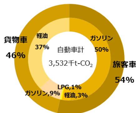
図 17 福島県の車種別燃料別二酸化炭素排出割合
