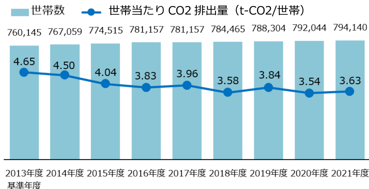
図 26 福島県の世帯数及び世帯当たり二酸化炭素排出量の推移
