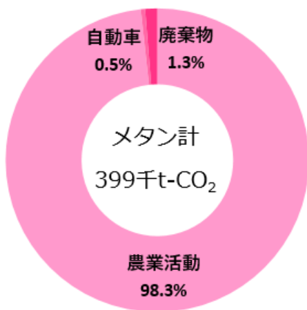
図 31 福島県のメタンの排出割合
