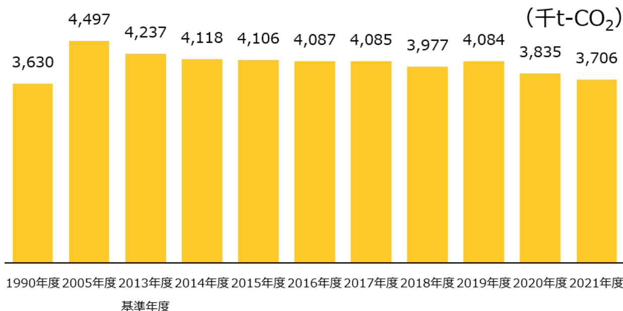
図 15 福島県の運輸部門の二酸化炭素排出量の推移
