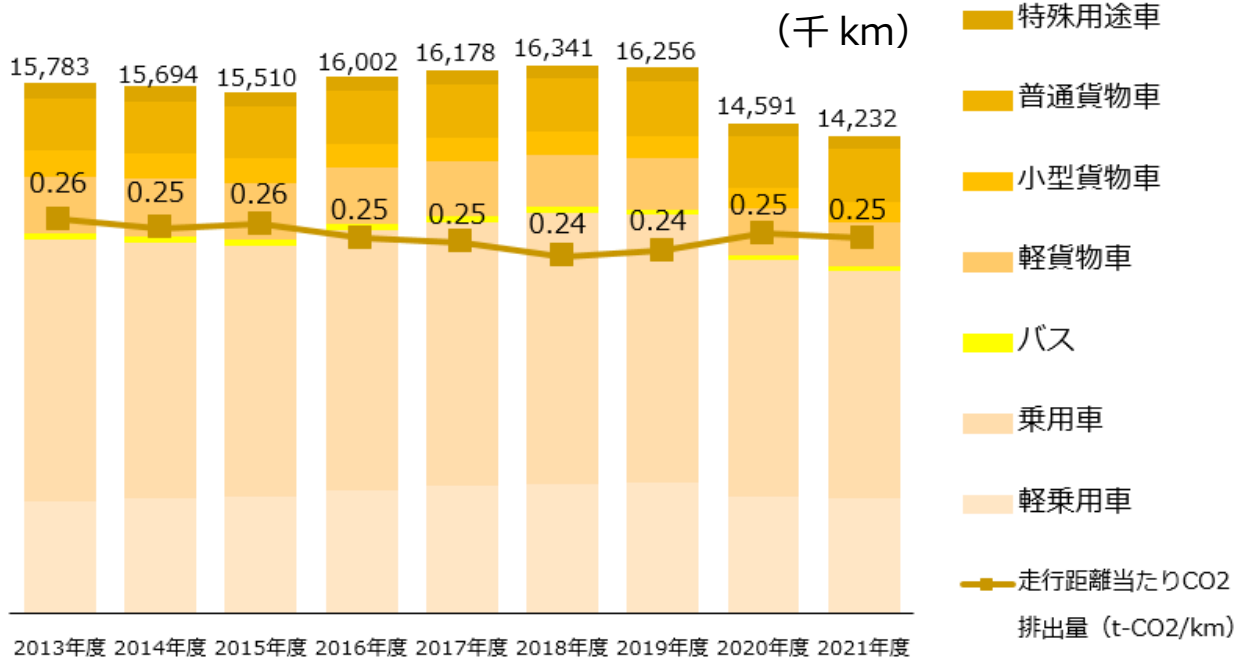
図 18 福島県の自動車車種別走行距離の推移
