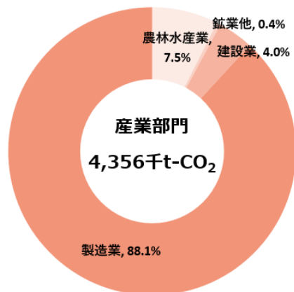
図 12 福島県の産業部門の業種別二酸化炭素排出割合
