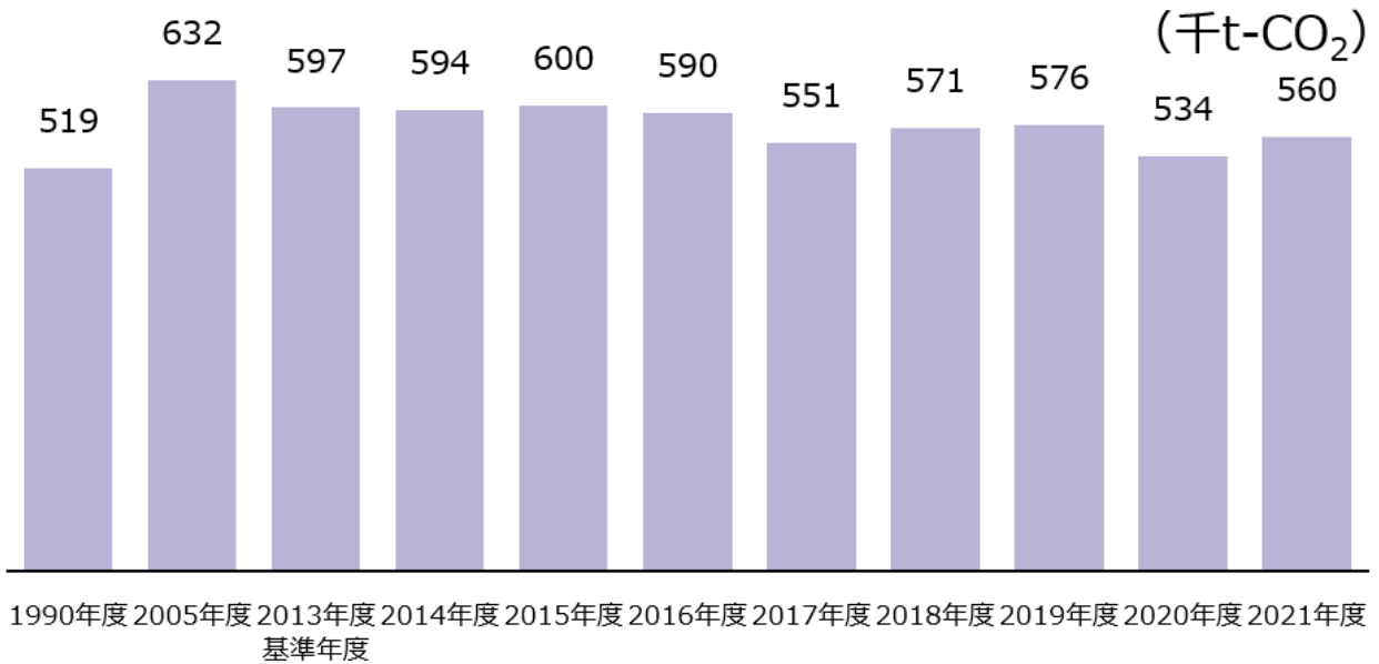
図 27 福島県の廃棄物部門の二酸化炭素排出量の推移
