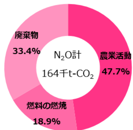
図 32 福島県の一酸化二窒素の排出割合
