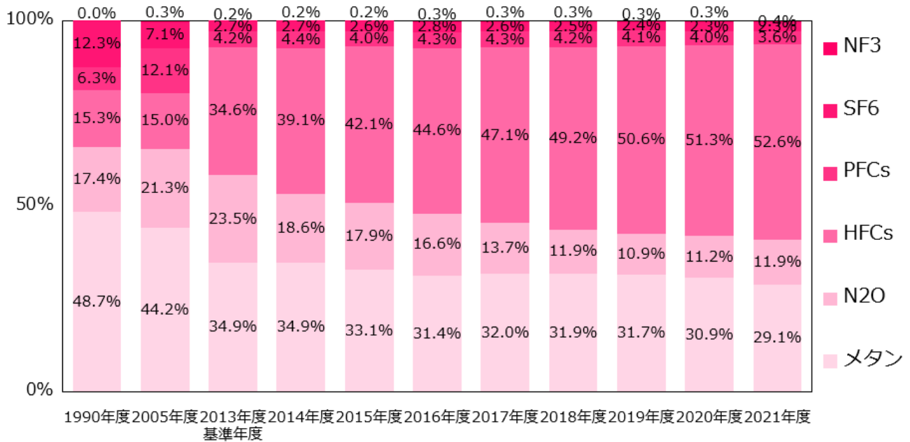
図 30 福島県のその他温室効果ガスの排出割合の推移
