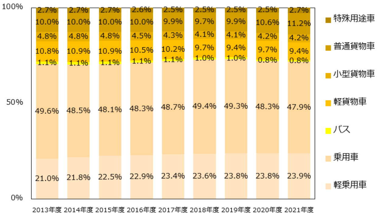
図 19 福島県の自動車車種別走行距離割合の推移
