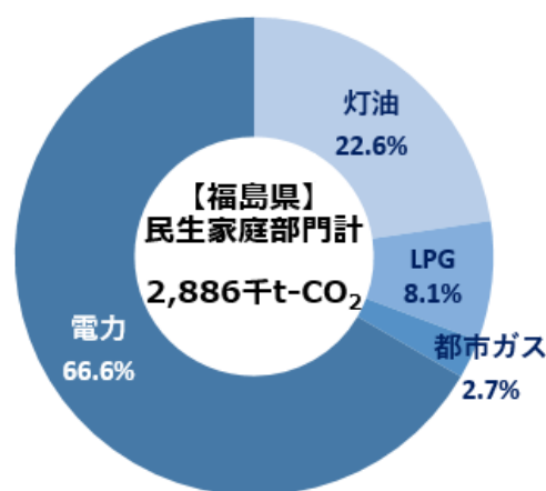
図 23 福島県の民生家庭部門のエネルギー別二酸化炭素排出割合
