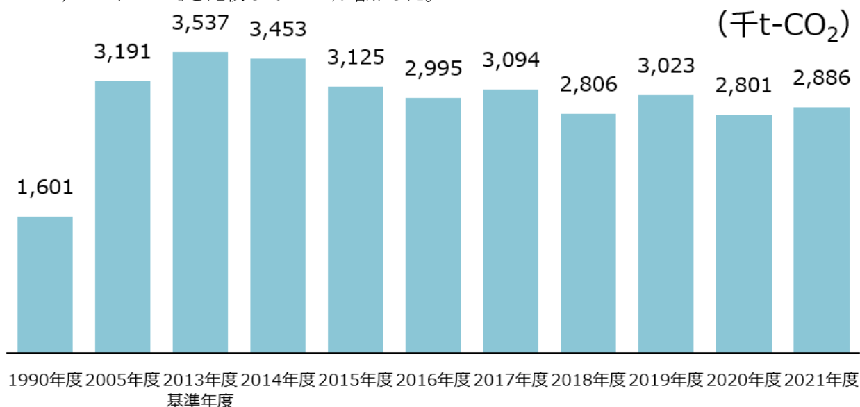
図 22 福島県の民生家庭部門の二酸化炭素排出量の推移
