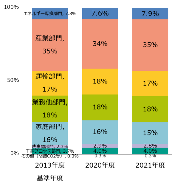
図 10 全国の部門別二酸化炭素排出割合
