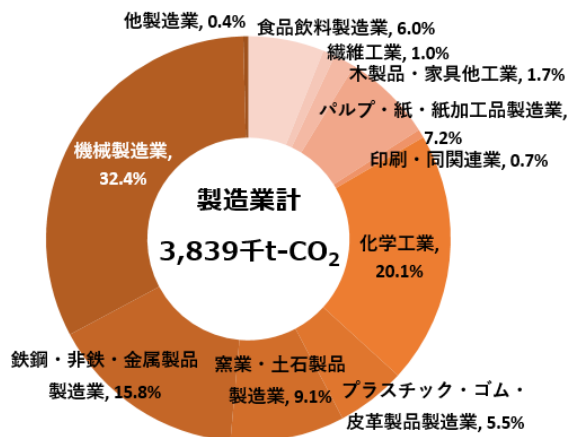
図 13 福島県の製造業の業種別二酸化炭素排出割合
