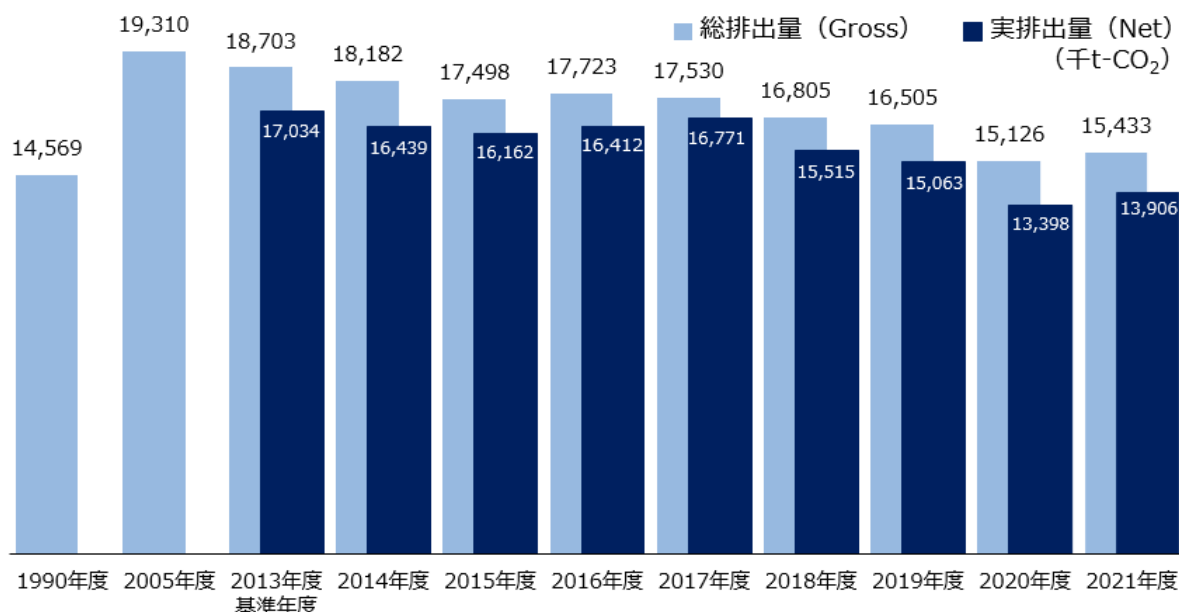
図 5 福島県の温室効果ガス排出量の推移
