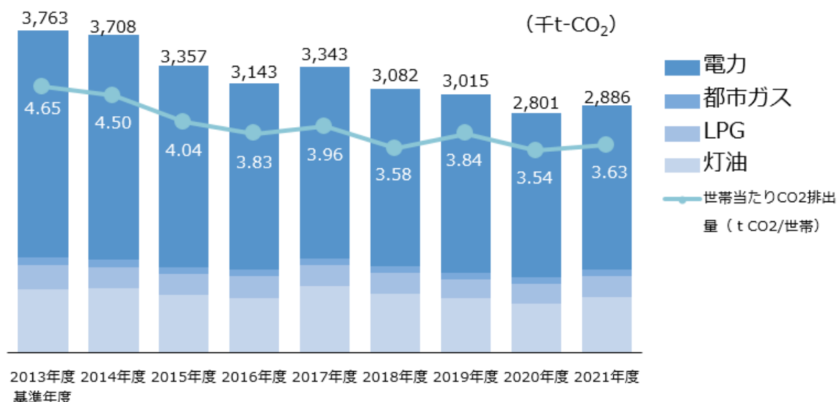
図 25 福島県の民生家庭部門のエネルギー別二酸化炭素排出量及び世帯当たり二酸化炭素排出量の推移
