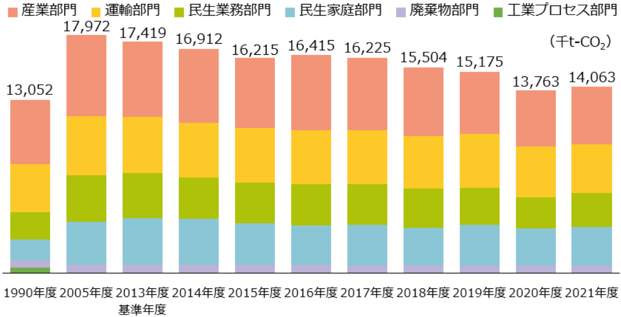
図 8 福島県の二酸化炭素排出量の推移
