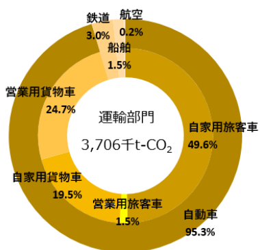
図 16 福島県の運輸部門の二酸化炭素排出割合
