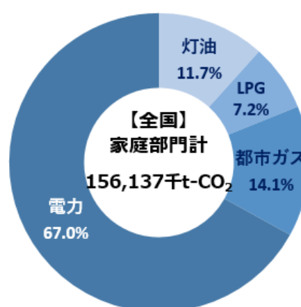
図 24 全国の家部門のエネルギー別二酸化炭素排出割合
