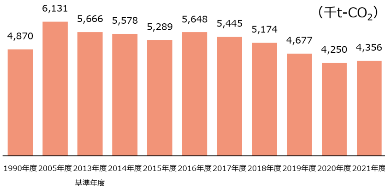
図 11 福島県の産業部門の二酸化炭素排出量の推移
