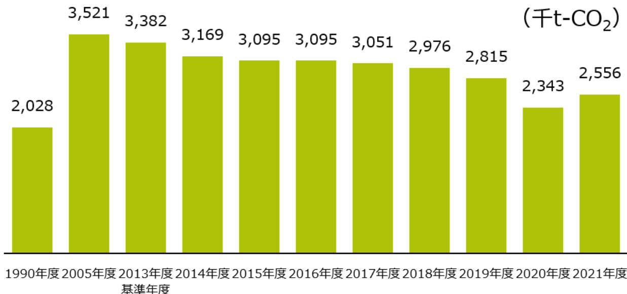
図 20 福島県の民生業務部門の二酸化炭素排出量の推移
