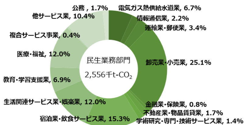
図 21 福島県の民生業務部門の業種別二酸化炭素排出割合
