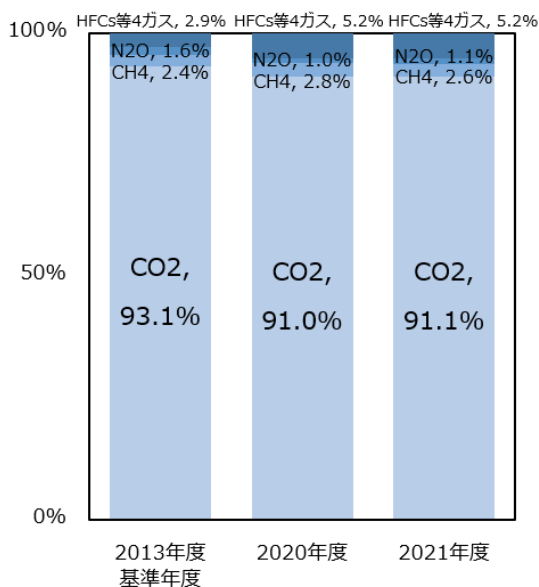
図 6 福島県の温室効果ガス排出割合
