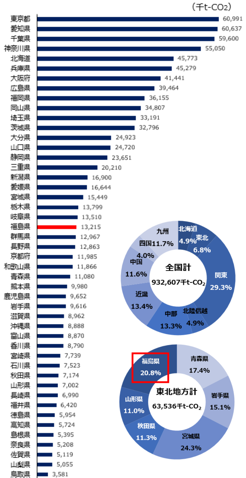
図 34 都道府県別二酸化炭素排出量推計結果 (2020 年度)
