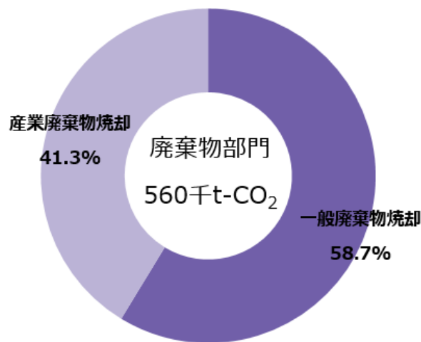
図 28 福島県の廃棄物部門の二酸化炭素排出割合
