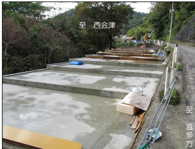
国道459号 堂山工区 (喜多方市)
