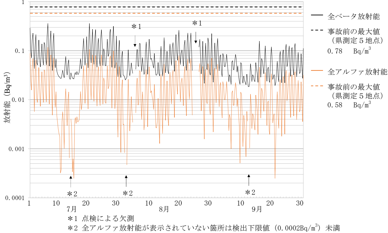
大気浮遊じんの全アルファ及び全ベータ放射能の推移 (6時間連続集じん・6時間放置後測定) 15 南相馬市萱浜 (令和7年7月1日～9月30日)
