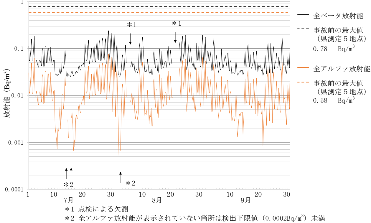
大気浮遊じんの全アルファ及び全ベータ放射能の推移 (6時間連続集じん・6時間放置後測定) 16 飯館村伊丹沢 (令和7年7月1日～9月30日)
