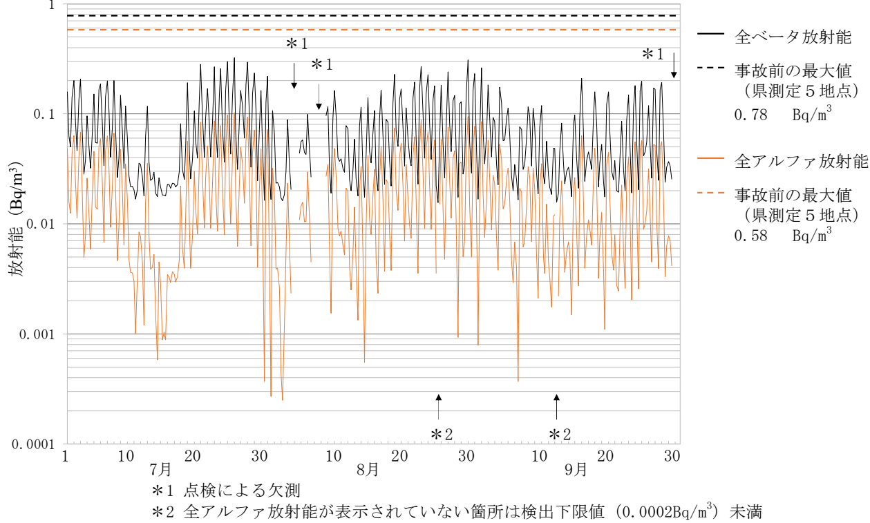
大気浮遊じんの全アルファ及び全ベータ放射能の推移 (6時間連続集じん・6時間放置後測定) 6 富岡町富岡 (令和7年7月1日～9月30日)
