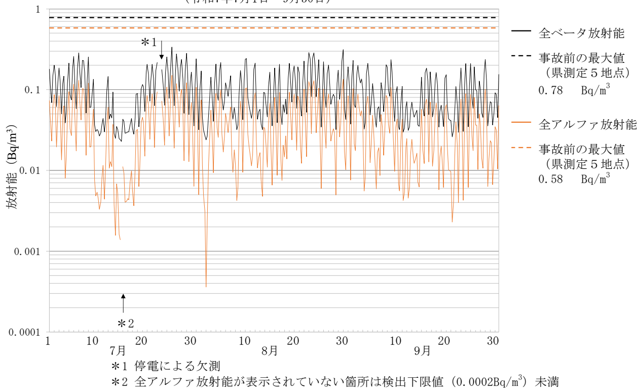
大気浮遊じんの全アルファ及び全ベータ放射能の推移 (6時間連続集じん・6時間放置後測定) 7 川内村下川内 (令和7年7月1日～9月30日)
