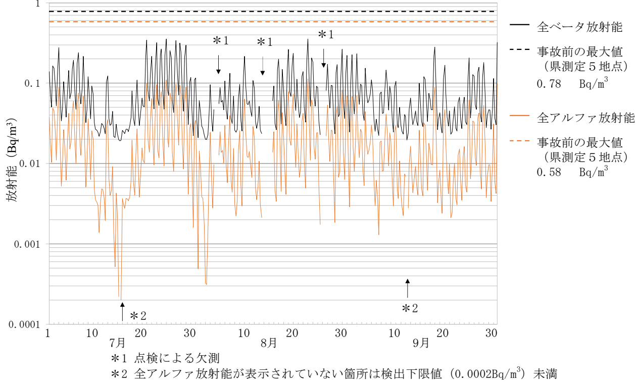
大気浮遊じんの全アルファ及び全ベータ放射能の推移 (6時間連続集じん・6時間放置後測定) 5 檜葉町繁岡 (令和7年7月1日～9月30日)
