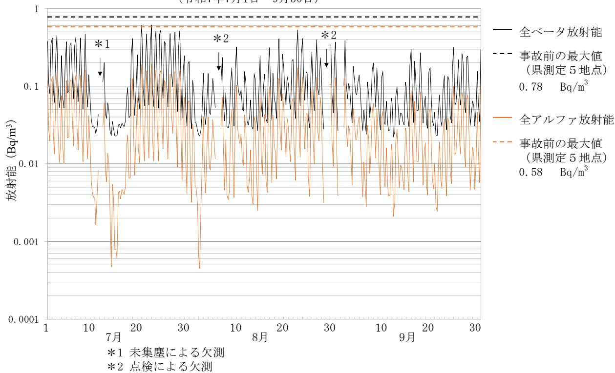
大気浮遊じんの全アルファ及び全ベータ放射能の推移 (6時間連続集じん・6時間放置後測定) 8 大熊町大野 (令和7年7月1日～9月30日)
