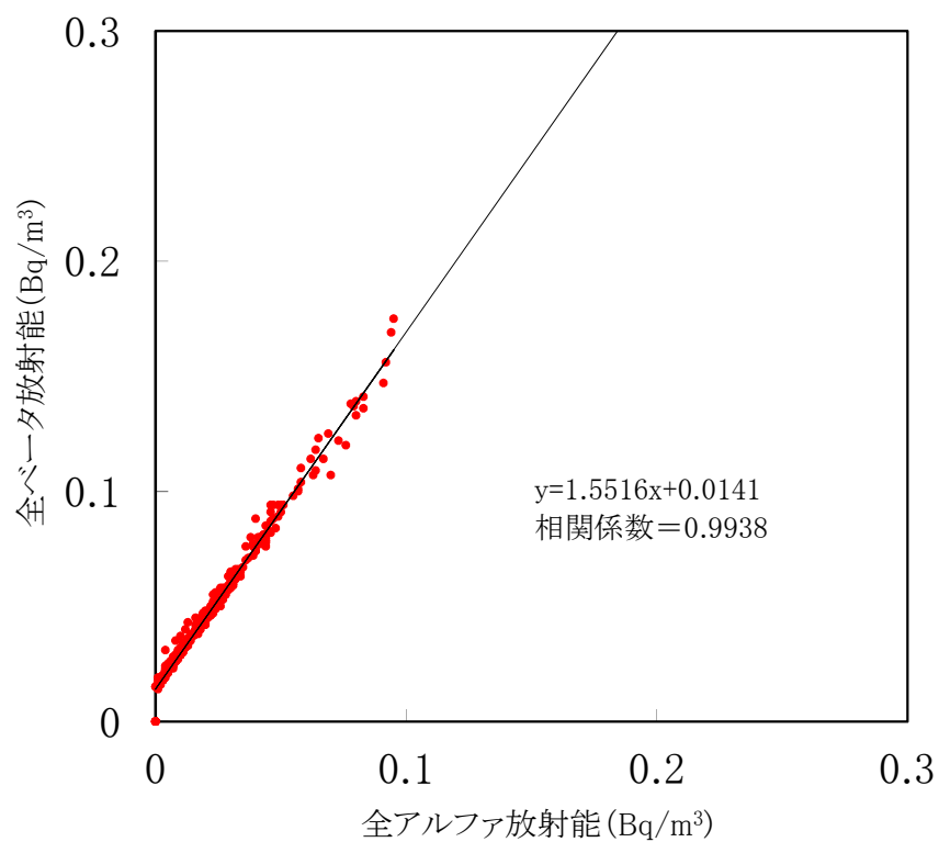
大気浮遊じんの全アルファ・全ベータ放射能の相関図 (MP-8) (令和7年7月～令和7年9月)
