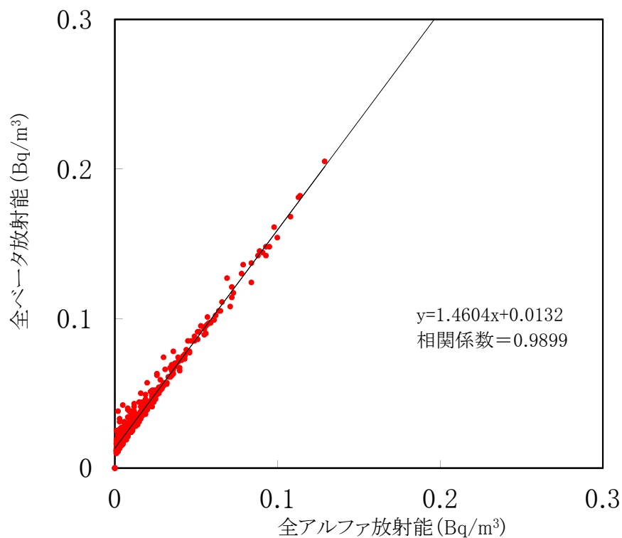
大気浮遊じんの全アルファ・全ベータ放射能の相関図 (MP-3) (令和7年7月～令和7年9月)
