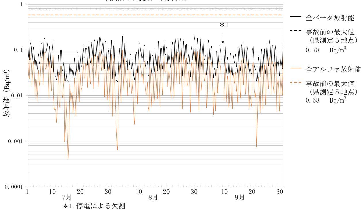
大気浮遊じんの全アルファ及び全ベータ放射能の推移 (6時間連続集じん・6時間放置後測定) 4 楡葉町木戸ダム (令和7年7月1日～9月30日)
