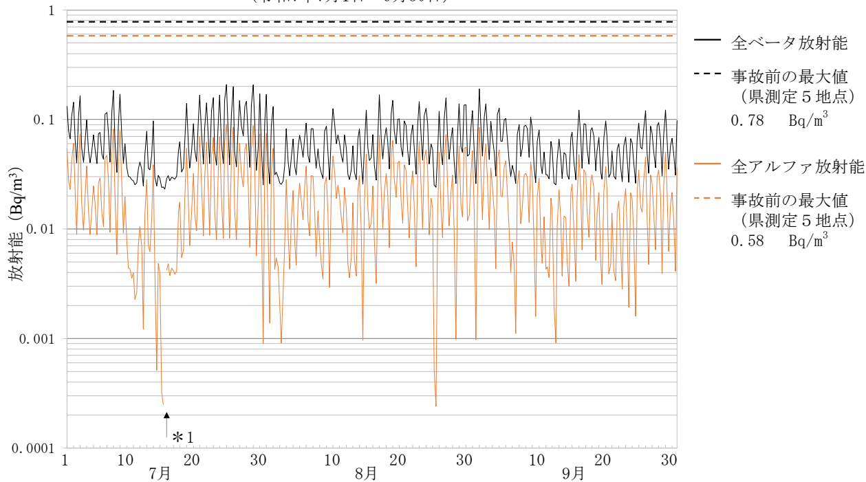
大気浮遊じんの全アルファ及び全ベータ放射能の推移 (6時間連続集じん・6時間放置後測定) 14 南相馬市泉沢 (令和7年7月1日～9月30日)
