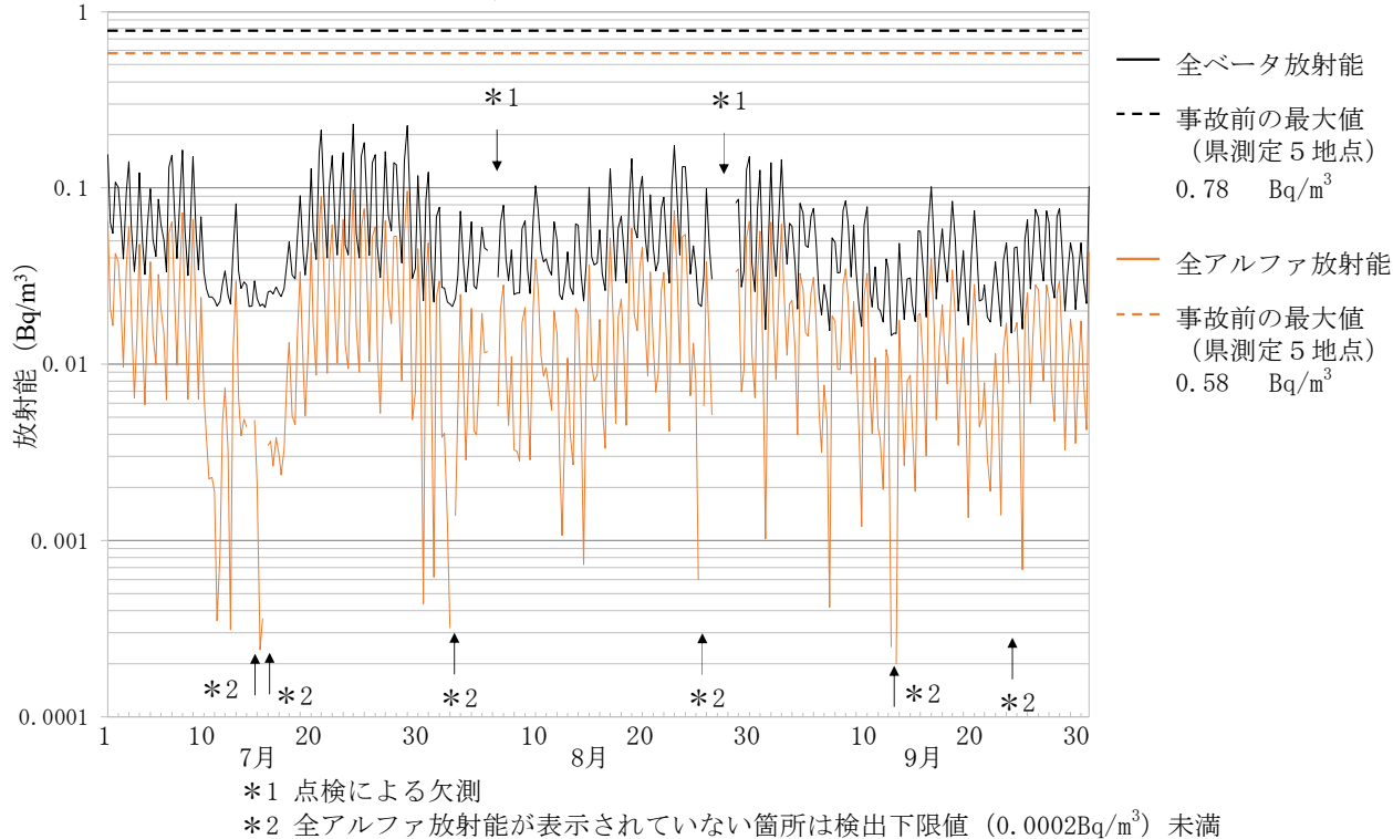
大気浮遊じんの全アルファ及び全ベータ放射能の推移 (6時間連続集じん・6時間放置後測定) 10 双葉町郡山 (令和7年7月1日～9月30日)
