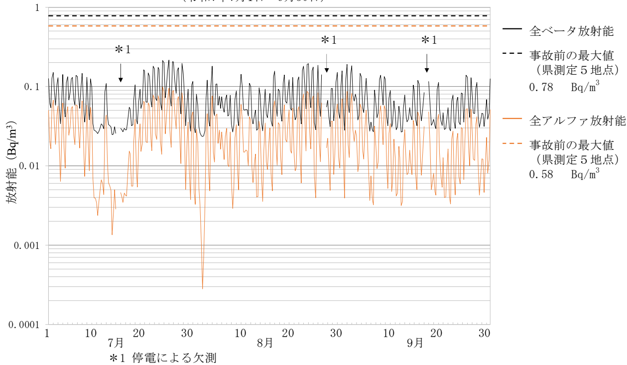
大気浮遊じんの全アルファ及び全ベータ放射能の推移 (6時間連続集じん・6時間放置後測定) 3 広野町小滝平 (令和7年7月1日～9月30日)
