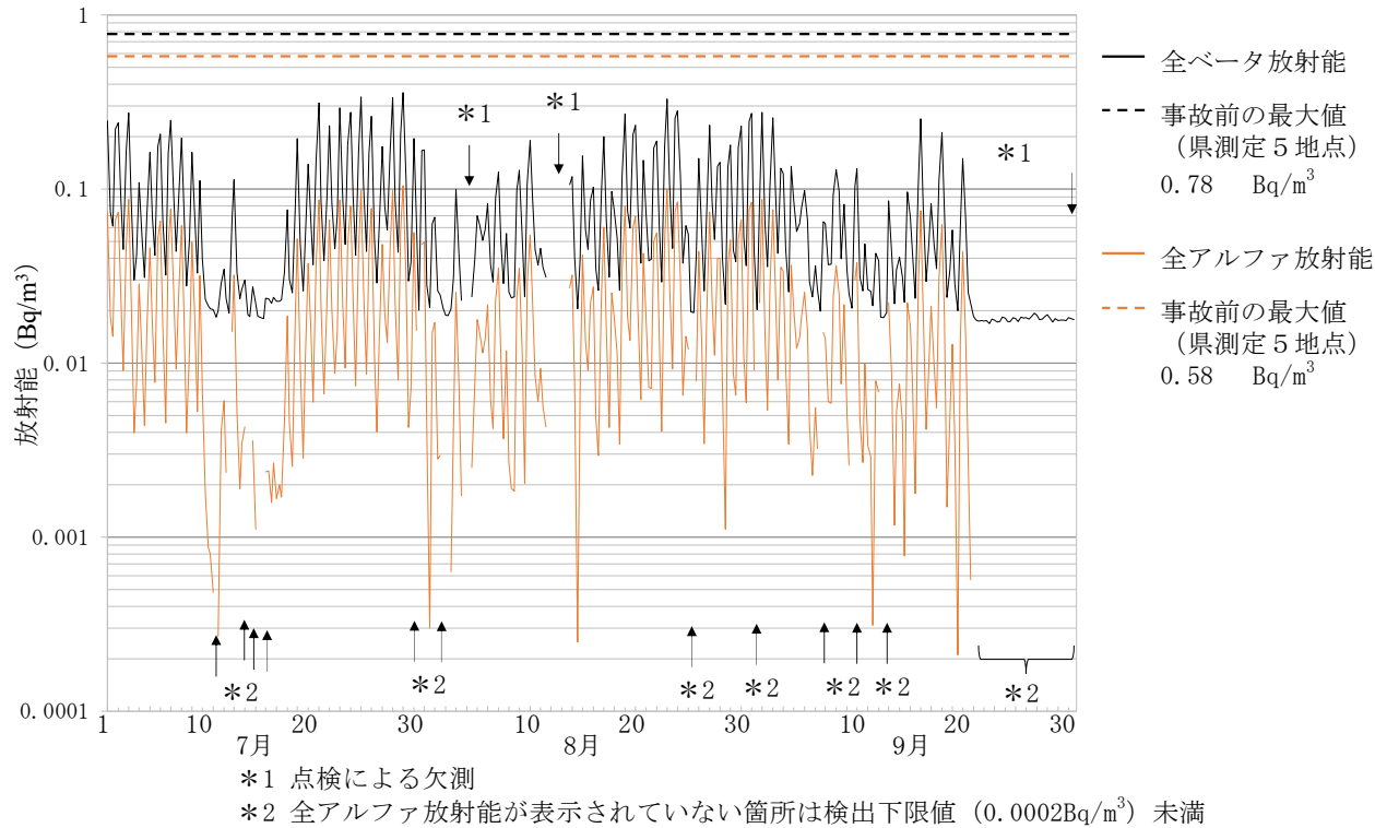
大気浮遊じんの全アルファ及び全ベータ放射能の推移 (6時間連続集じん・6時間放置後測定) 9 大熊町夫沢 (令和7年7月1日～9月30日)
