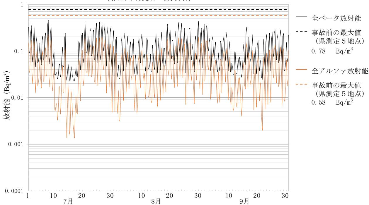
大気浮遊じんの全アルファ及び全ベータ放射能の推移 (6時間連続集じん・6時間放置後測定) 13 葛尾村夏湯 (令和7年7月1日～9月30日)
