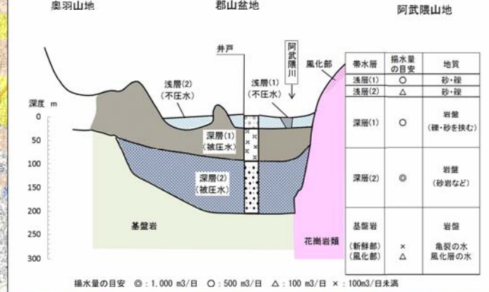
水理地質断面模式図
