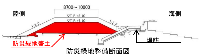
防災緑地整備断面図
