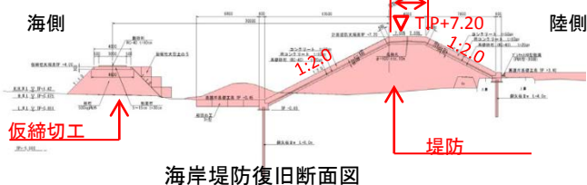
海岸堤防復旧断面図
