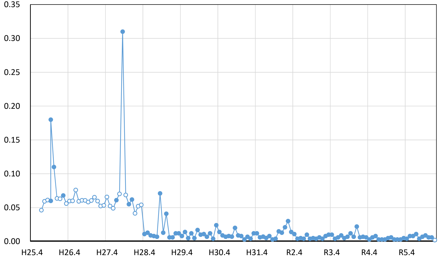
(5) 夫沢・熊川沖2km セシウム-137濃度の推移
