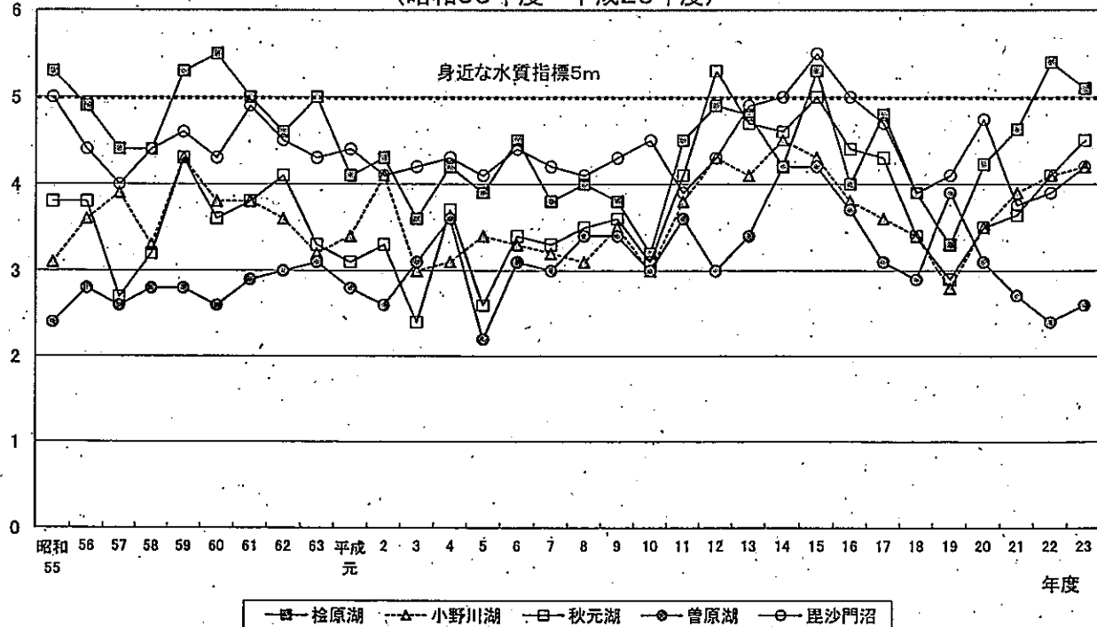
透明度 (m) 裏磐梯湖沼の透明度(年間平均値)の経年変化 (昭和55年度～平成23年度)
