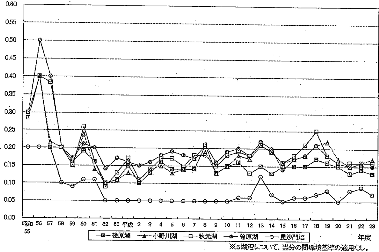
裏磐梯湖沼の全窒素(表層年間平均)の経年変化 (昭和55年度～平成23年度)
