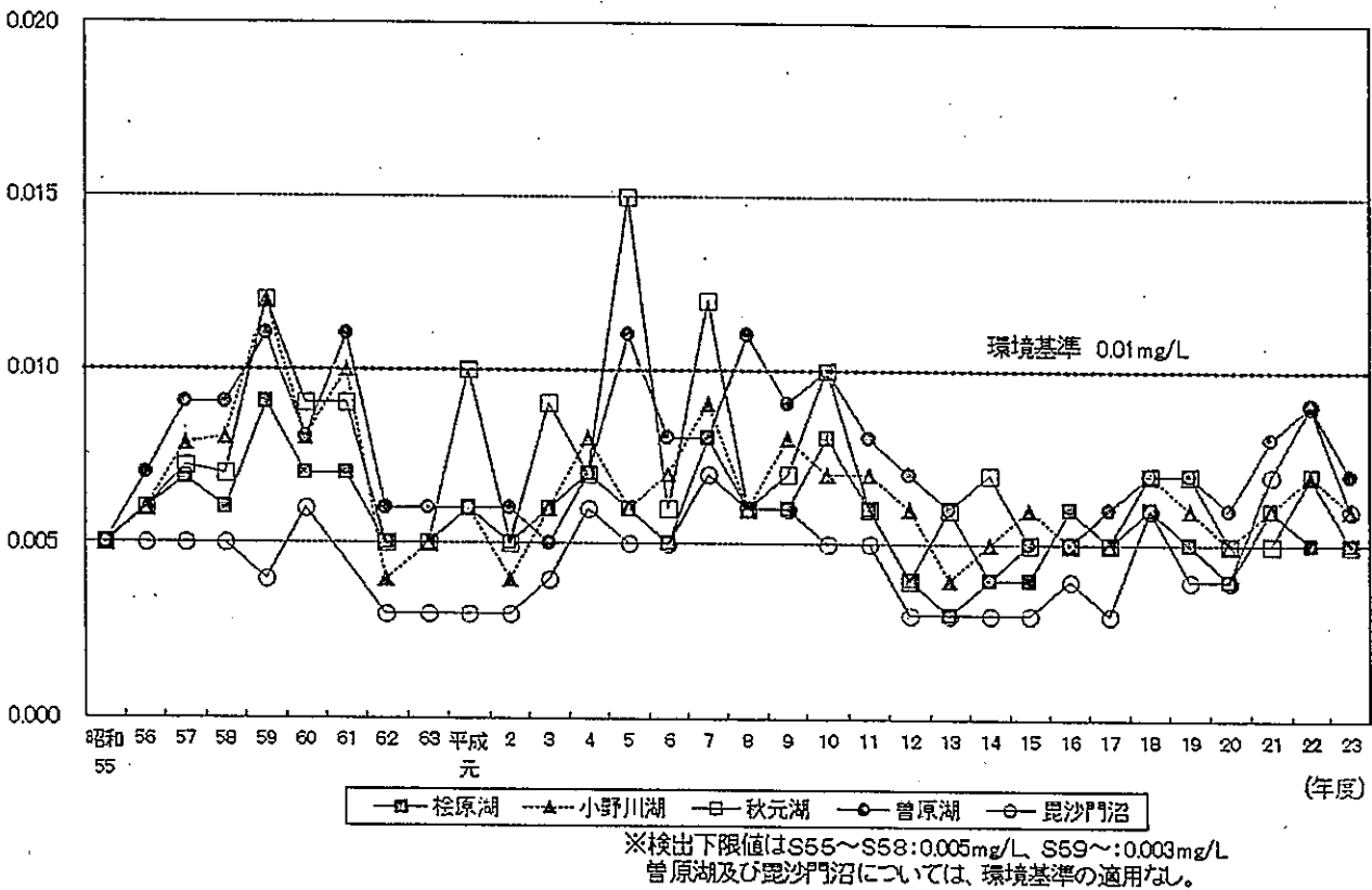
裏磐梯湖沼の全りん(表層年間平均)の経年変化 (昭和55年度～平成23年度)
