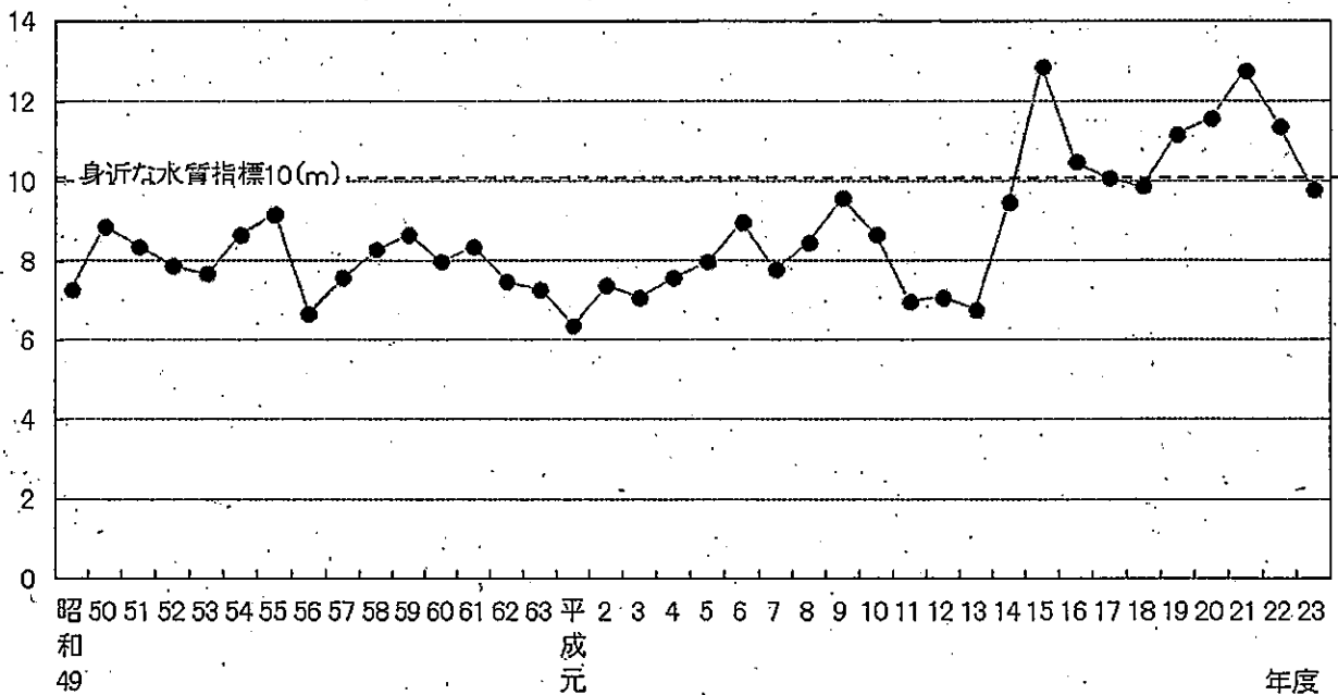
透明度(m) 猪苗代湖の透明度(年間平均値)の経年変化
