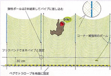
鳥獣害防止用簡易ネット柵(詳細図)
