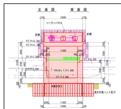
【水門一般図】
