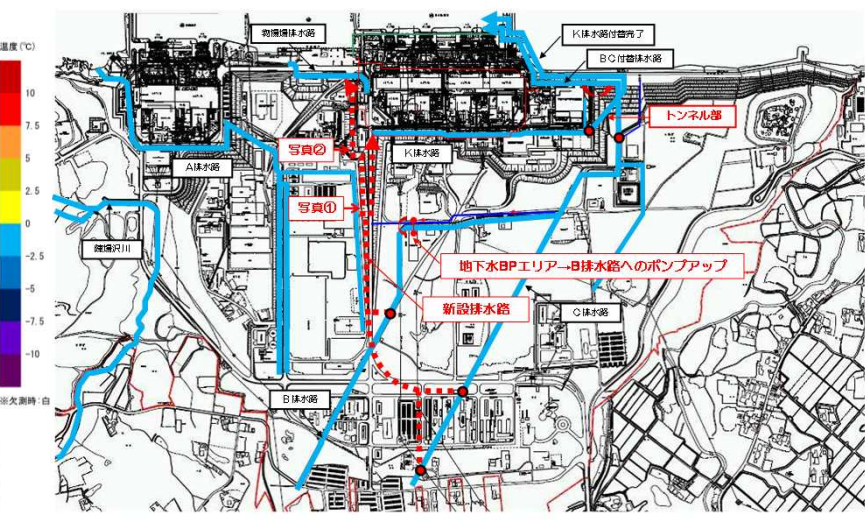
新設排水路の設置
