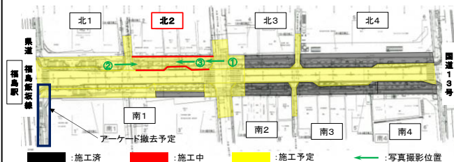
施工箇所図
