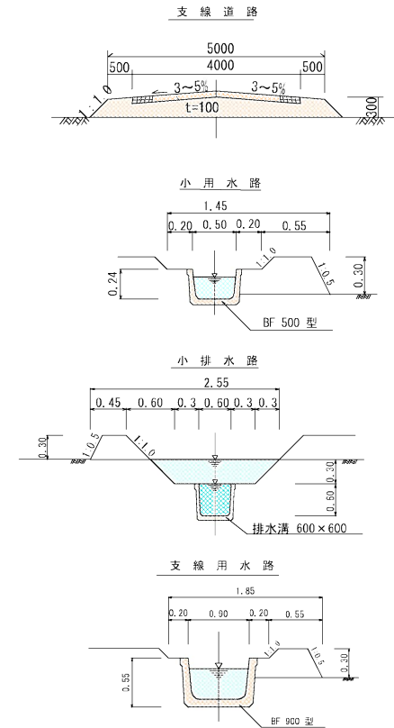
標準構造図
