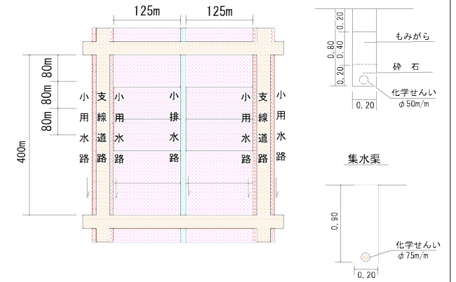
標準構造図
