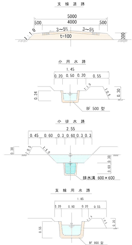
標準構造図
