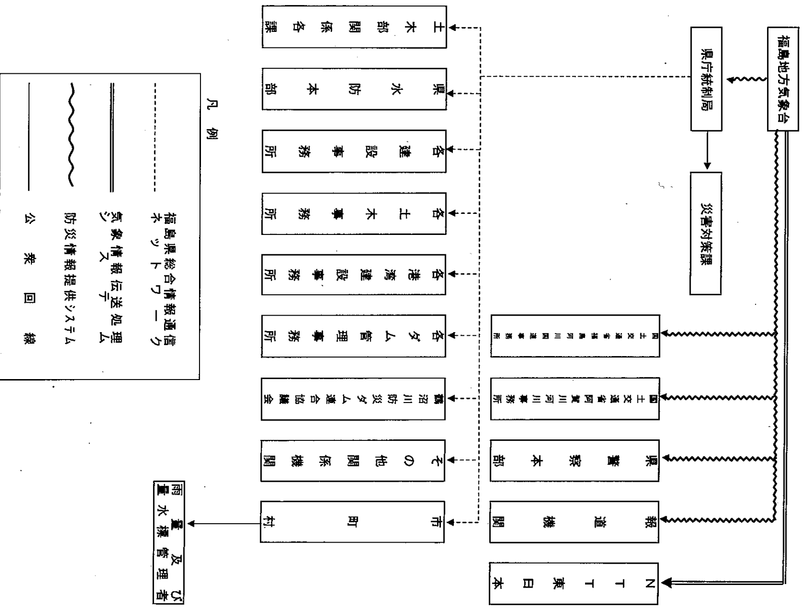
水防用気象予警報伝達系統図
