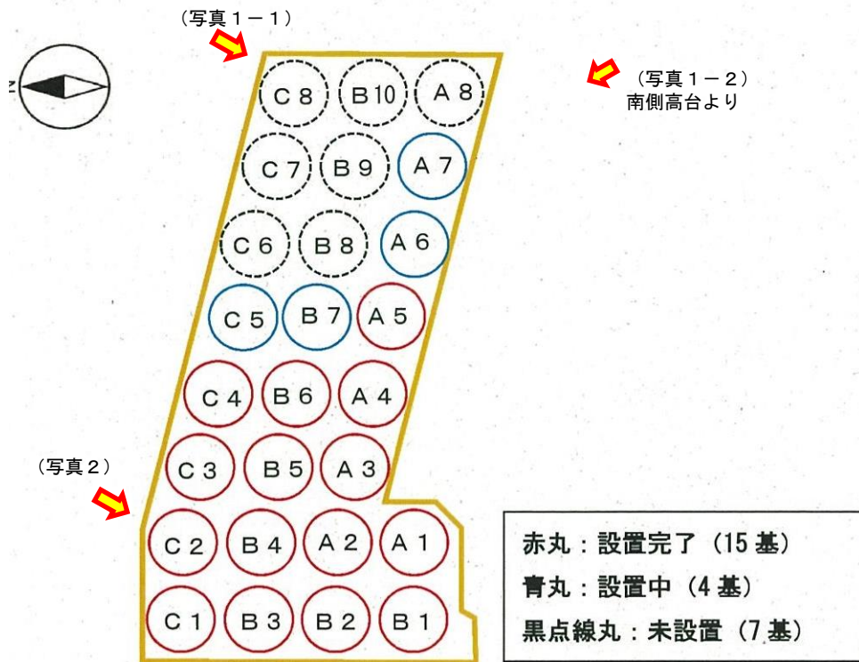
図2 G4南タンクエリア配置図
