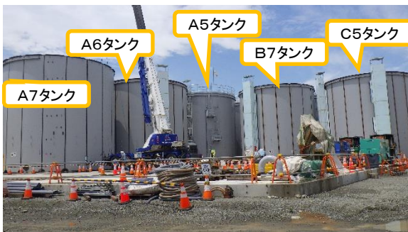
(写真1-1) G4南タンクエリアの状況① (北東側から撮影)
