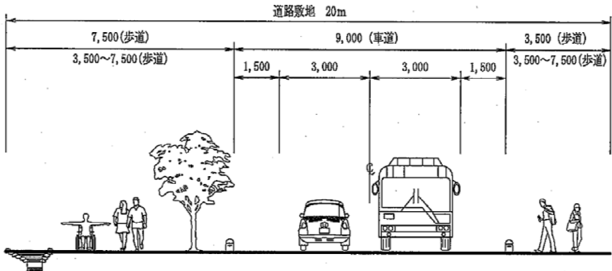
ワークショップにより提案された断面構成の基本的な考え方
