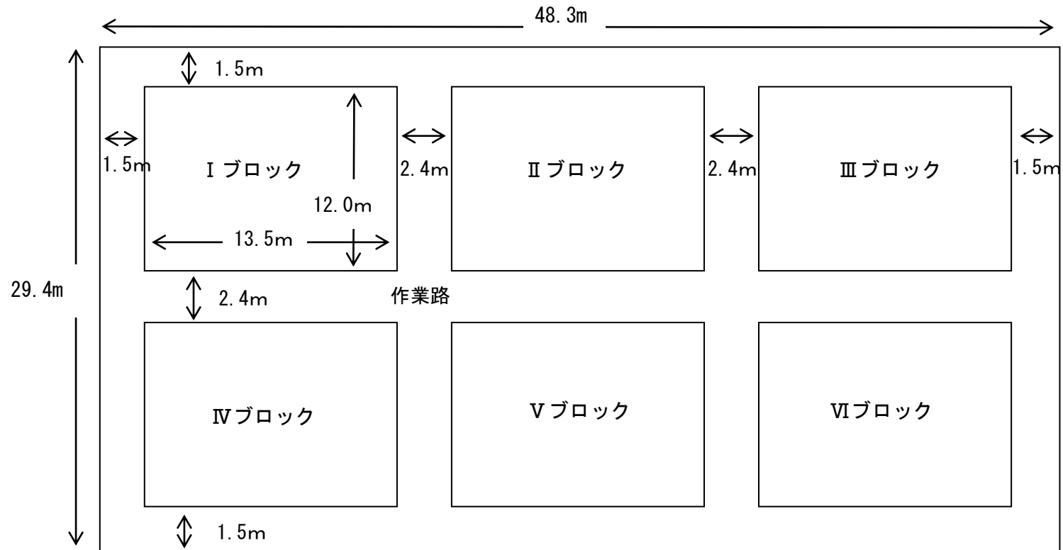
○ スギミニチュア採種園全体の設計図
