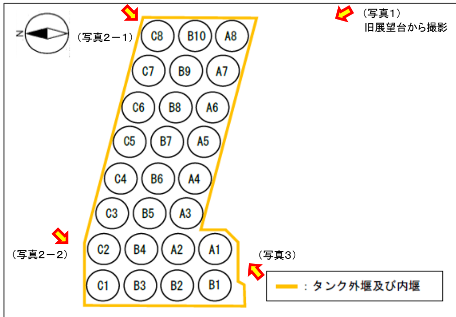
(図2) G4南タンクエリア配置図
