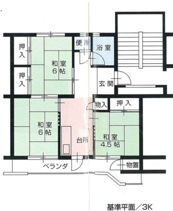
【間取り】
