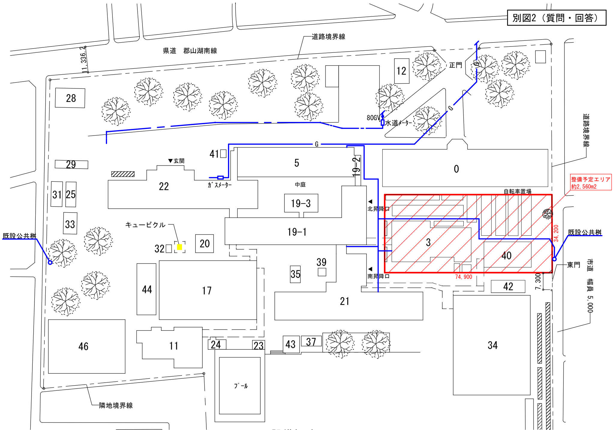
設備概略図
