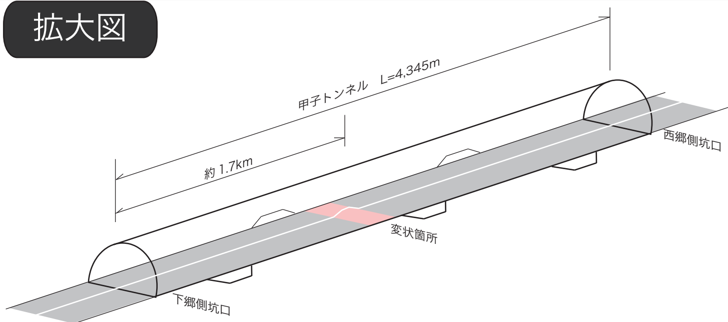
片側交互通行規制概要図
