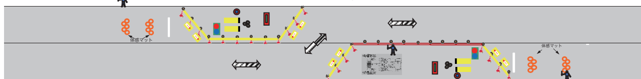
片側交互通行規制概要図
