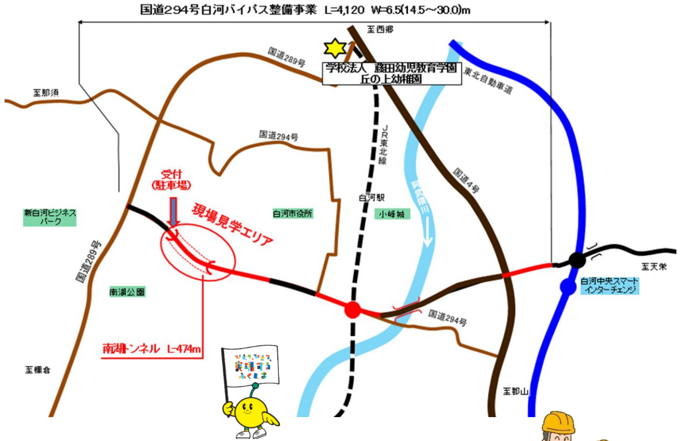
南湖トンネル 延長 L=474.0m 幅員 W=6.5(14.5)m
