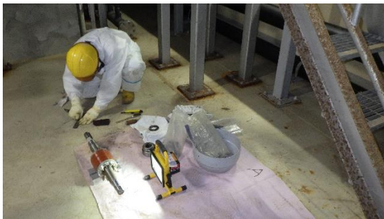
(写真 3 - 2) 2号機タービン建屋内炉注水ポンプ の定期点検の状況
