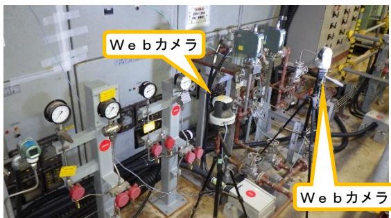
(写真2-1) 1号機室素封入設備の状況①
