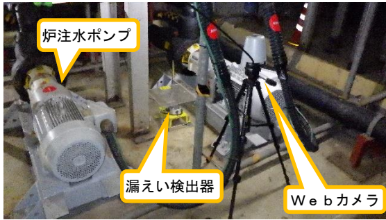
(写真5) 3号機タービン建屋内炉注水ポンプ の状況
