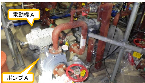
(写真1) ポンプから取外しされた電動機の状況 (1号機タービン建屋内炉注水ポンプAの例)
