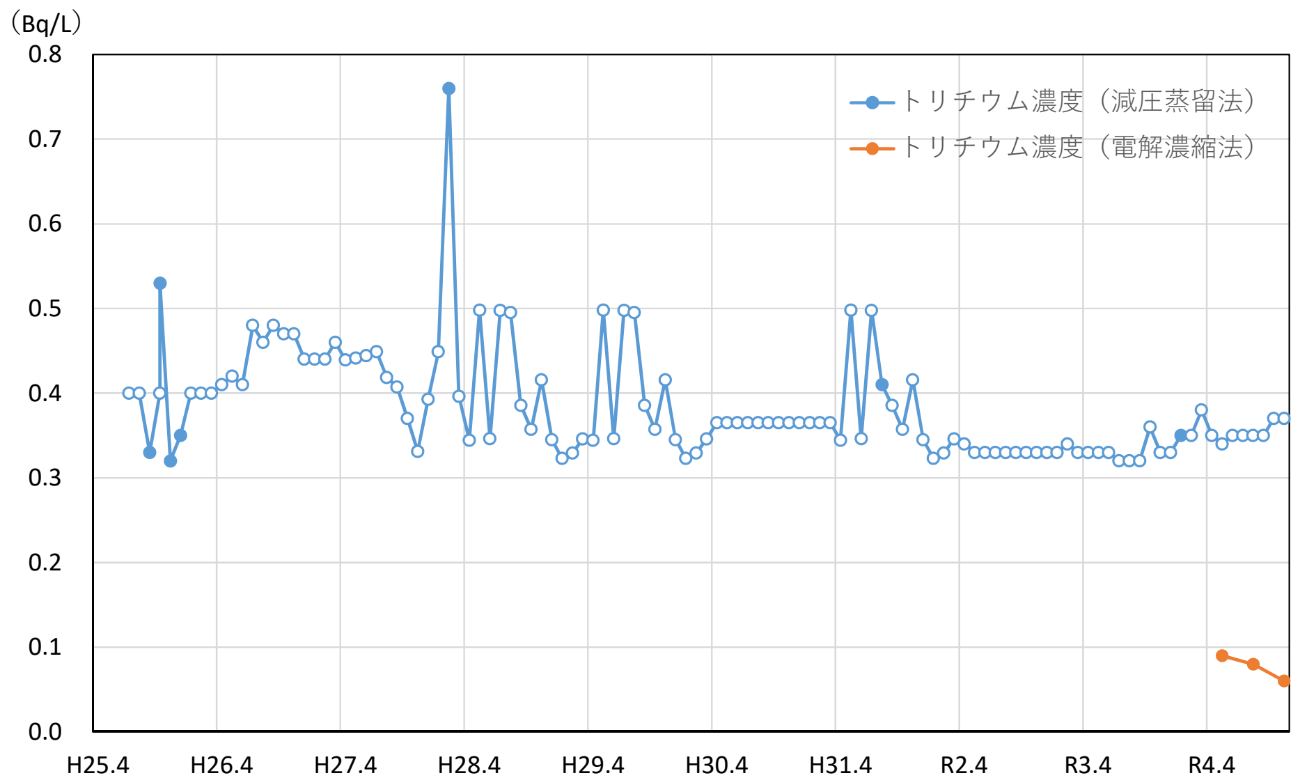
⑤ 夫沢・熊川沖2km トリチウム濃度の推移
