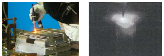
<実験例2> 左：TIG溶接、右：溶融池観察（MAG溶接）
