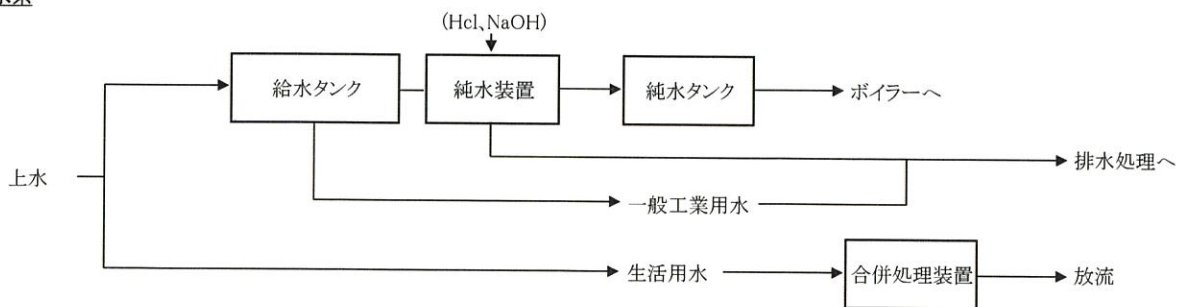
【図-4】 用水系
