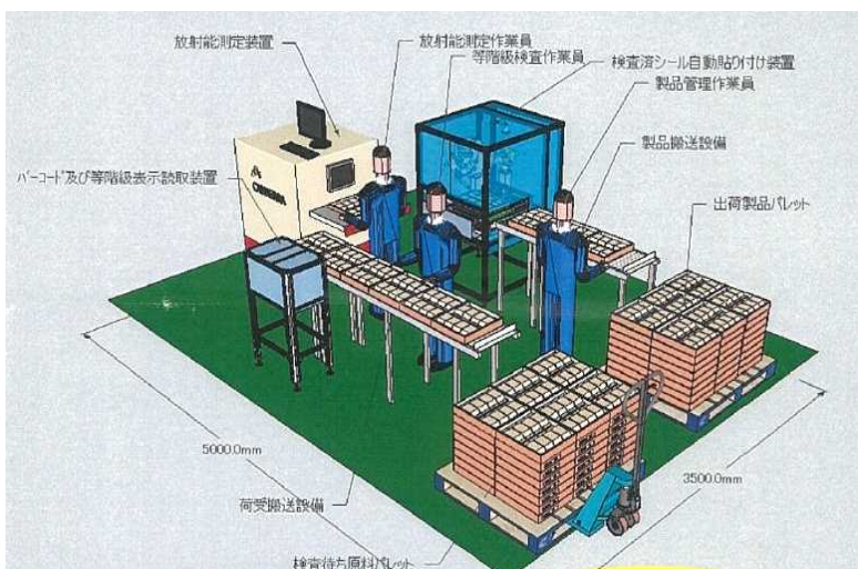
図1 あんぽ柿出荷箱の非破壊検査のイメージ
