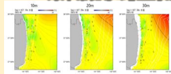
水深別水温
