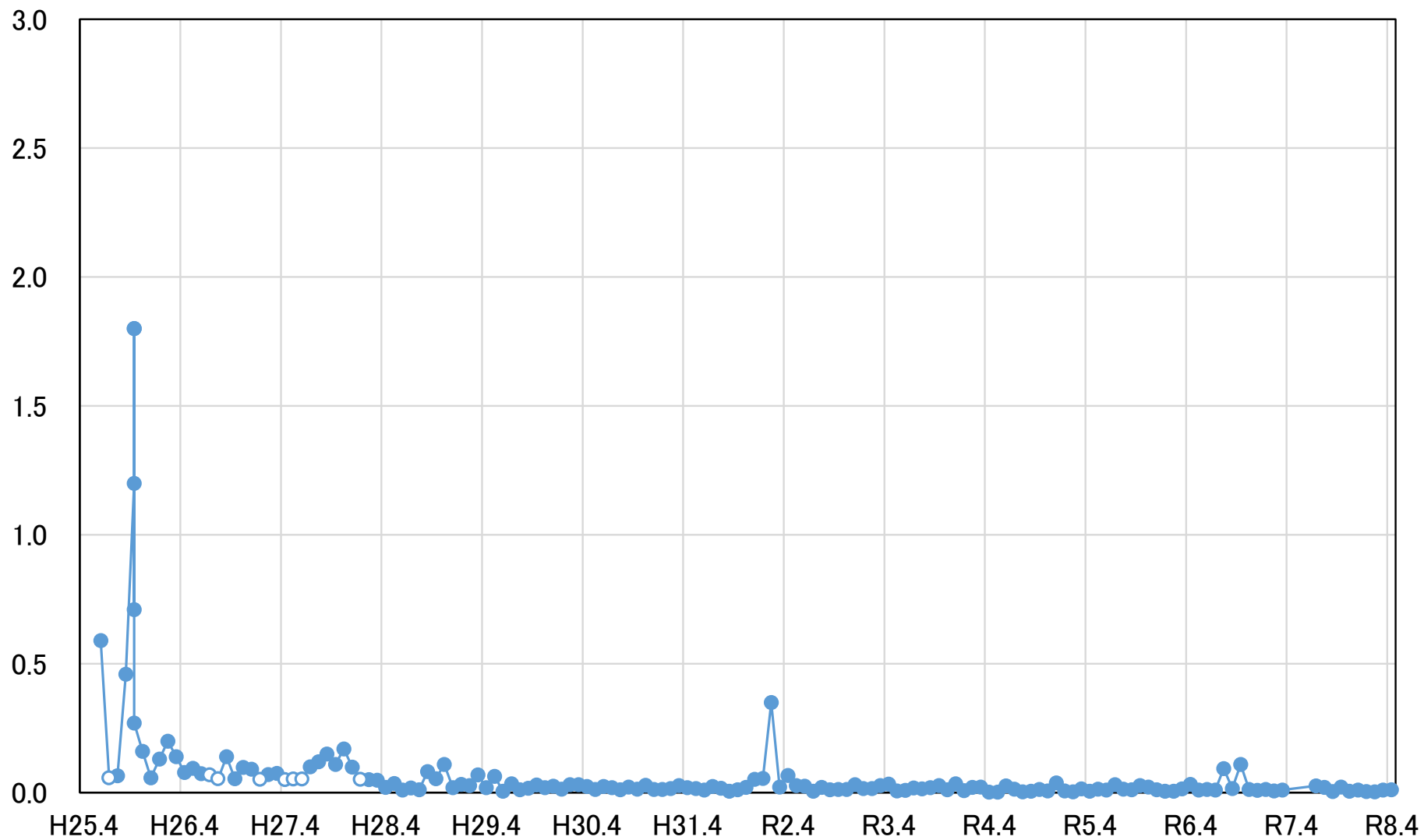
(1)南放水口 セシウム-137濃度の推移
