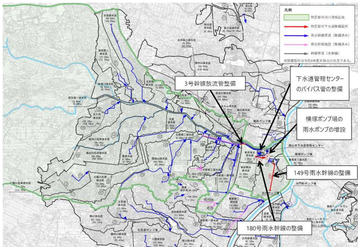
図 6.1 逢瀬川特定都市河川流域 特定都市下水道整備位置図
