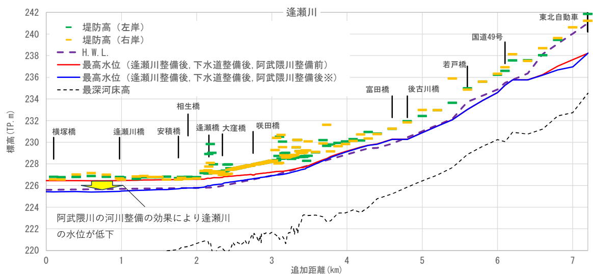
図 13.4 阿武隈川の整備前後における逢瀬川の水位縦断面図
