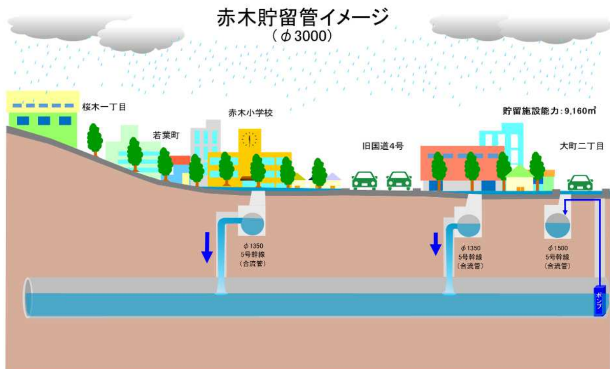
図 1.11 郡山市ゲリラ豪雨対策 9 年プランの対策イメージ (赤木貯留管)
