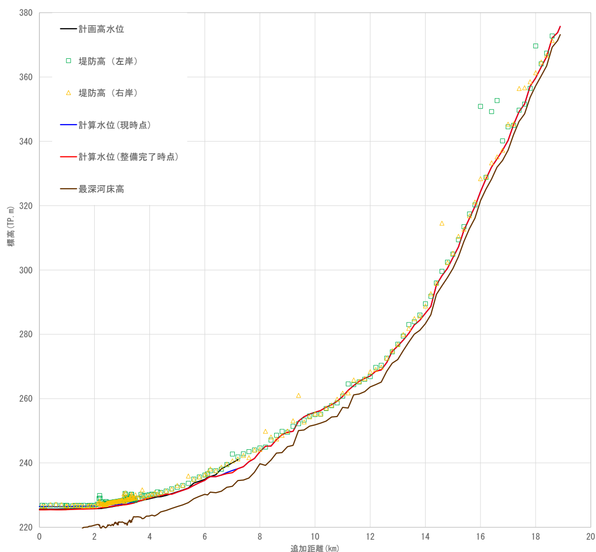
図 4.1 逢瀬川水位縦断図（福島県）
