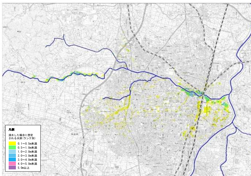
図 3.1 都市浸水想定
