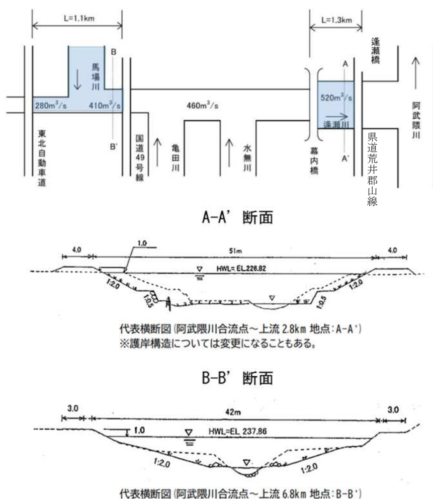
図 4.2 河川整備範囲
