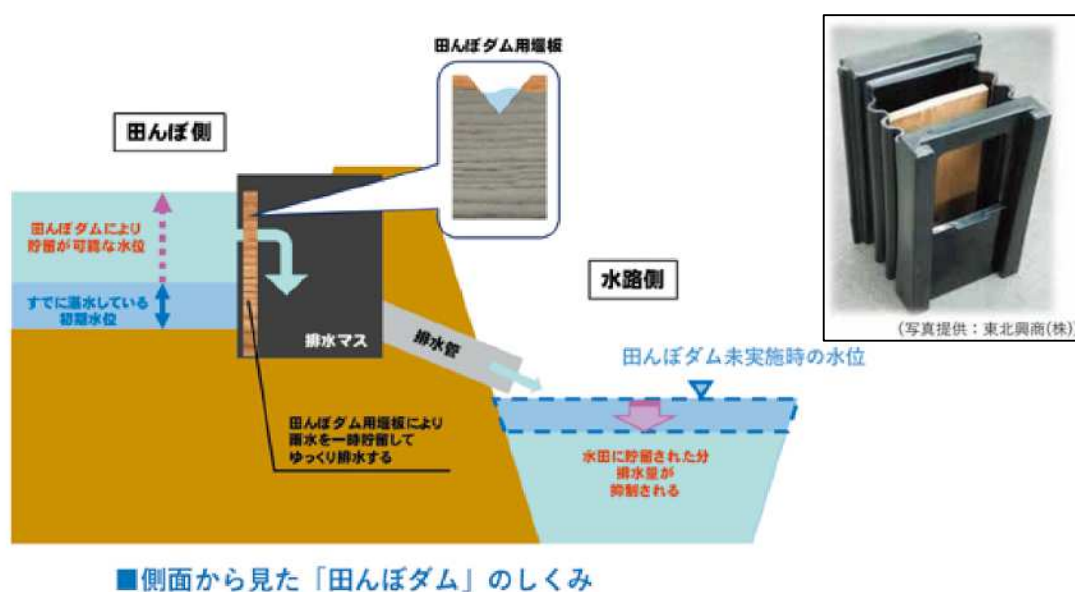
出典：田んぼダム技術マニュアル 令和8年3月 福島県農林水産部農村振興課 図 7.3 水田の活用（「田んぼダム」）の仕組み
