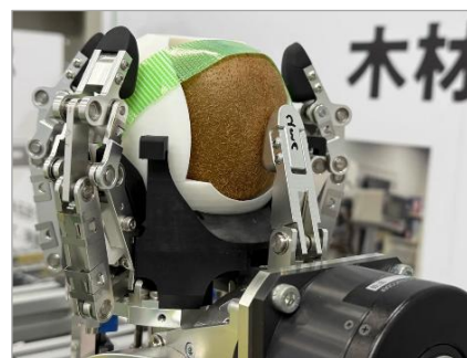
ロボットハンドのデモ実演
